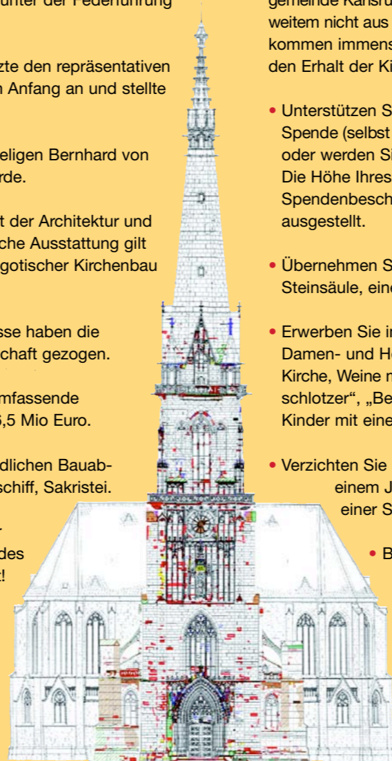
Schadenskartierung der unteren Turmhälfte und des Langhauses, Stand Dezember 2005
